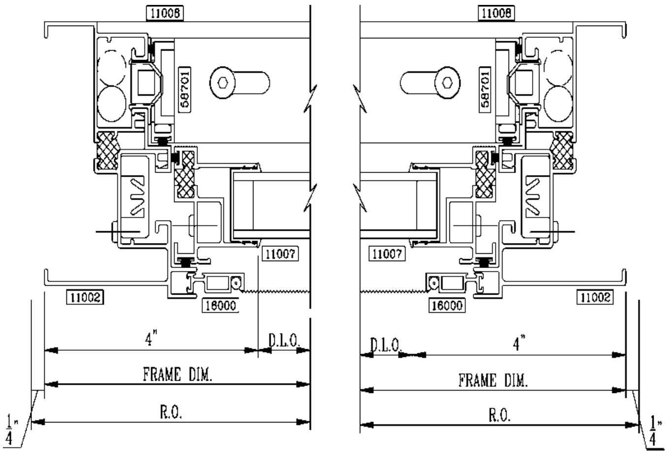
4 LEFT JAMB DOUBLE HUNG
