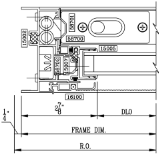
Left Jamb Double Hung
