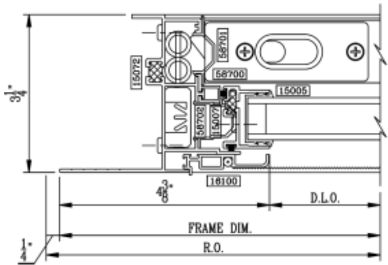
6 Flanged Jamb DH
