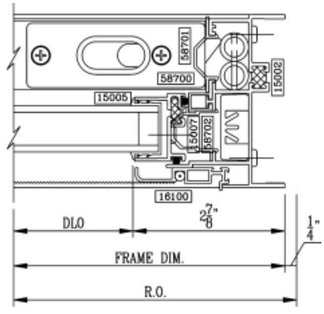
Right Jamb Double Hung
