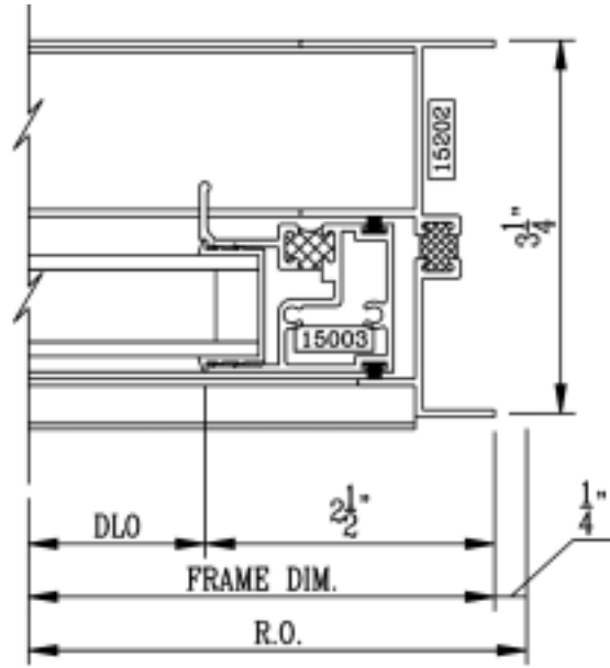
Right Jamb Slider
