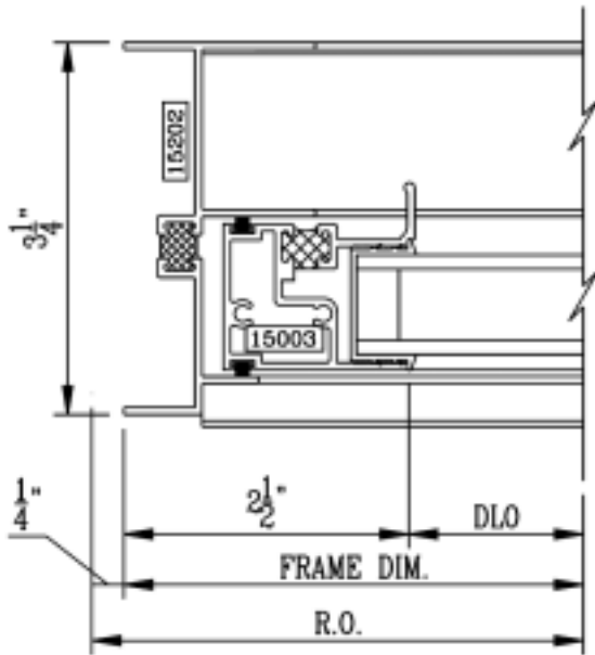
Left Jamb Slider
