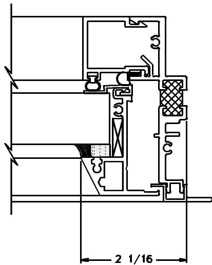
⑥ RIGHT JAMB P7500
