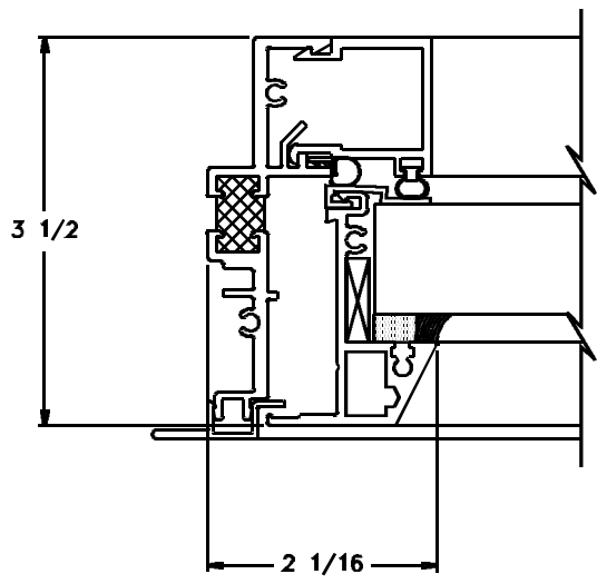
④ LEFT JAMB P7500
